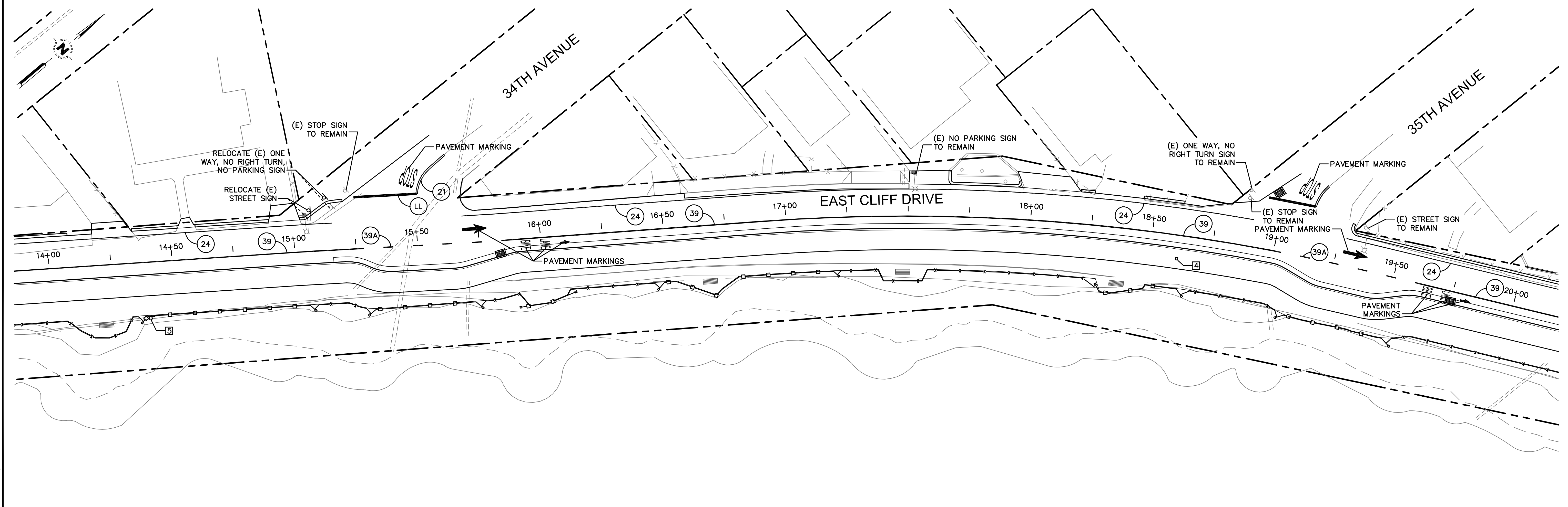
STRIPING AND SIGNAGE PLAN STA 10+00 - 20+00 SCALE: 1" = 20'
